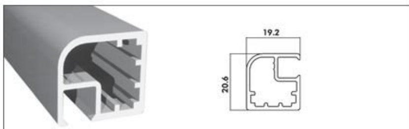
■ SAS 005 keretprofil
