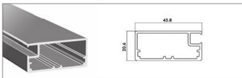
■ SAS 006 keretprofil
